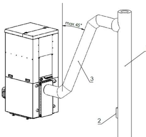
Rysunek 15 - Podłączenie do instalacji kominowej – pochylone 1 – Przewód kominowy; 2 – Wyczystka kominą; 3 – Zaizolowane podłączenie do kominą
