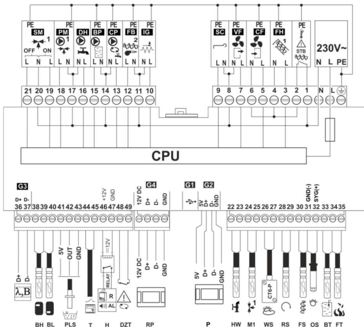
Rysunek 21 - Schemat połączeń elektrycznych regulatora: λ – moduł sondy Lambda, B – moduł do obsługi dodatkowych obiegów grzewczych, BH – czujnik temperatury bufora górny typu CT4, BL – czujnik temperatury bufora dolny typu CT4, PLS – czujnik poziomu paliwa, T – termostat pokojowy (zwierno-rozwierny), H – wyjście napięciowe do sterowania kotłem rezerwowym R lub do sygnalizacji alarmów AL , RELAY – przekaźnik 12VDC, DZT – czujnik otwarcia drzwi kotła, RP – panel pokojowy ecoSTER TOUCH z funkcją termostatu pokojowego, P – panel sterujący, HW – czujnik temperatury CWU typu CT4, M1 – czujnik temperatury obiegu regulowanego (mieszacza 1) typu CT4, WS – pogodowy czujnik temperatury typu CT6-P, RS – czujnik temperatury wody powracającej do kotła typu CT4, FS – czujnik temperatury podajnika typu CT4, OS – optyczny czujnik jasności płomienia, BT – czujnik temperatury kotła typu CT4, FT – czujnik temperatury spalin typu CT2S, L N PE – zasilanie sieciowe 230V~, CPU – sterowanie, STB – wejście do ogranicznika temperatury bezpieczeństwa, FH – podajnik główny, CF – wentylator nadmuchiwy palnika, VF – wentylator wyciągowy, SC – silnik obrotowy czyszczenia palnika, IG – zapalarka, FB – podajnik palnika, CP – pompa cyrkulacji CWU, BP – pompa kotła, DH – pompa CWU, PM – pompa mieszacza 1, SM – siłownik mieszacza 1.
