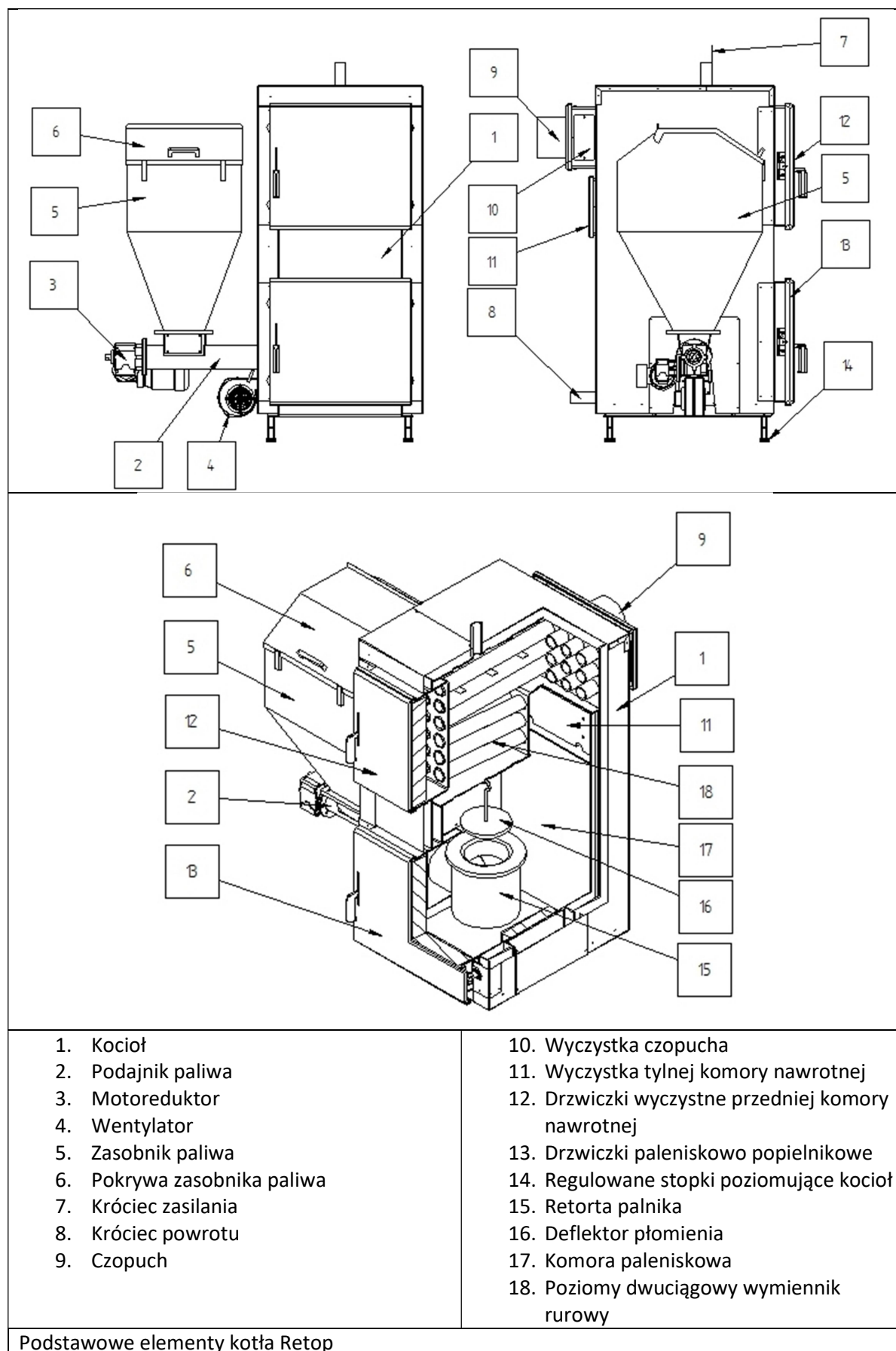
Rys.2. Kocioł „RETOP”
