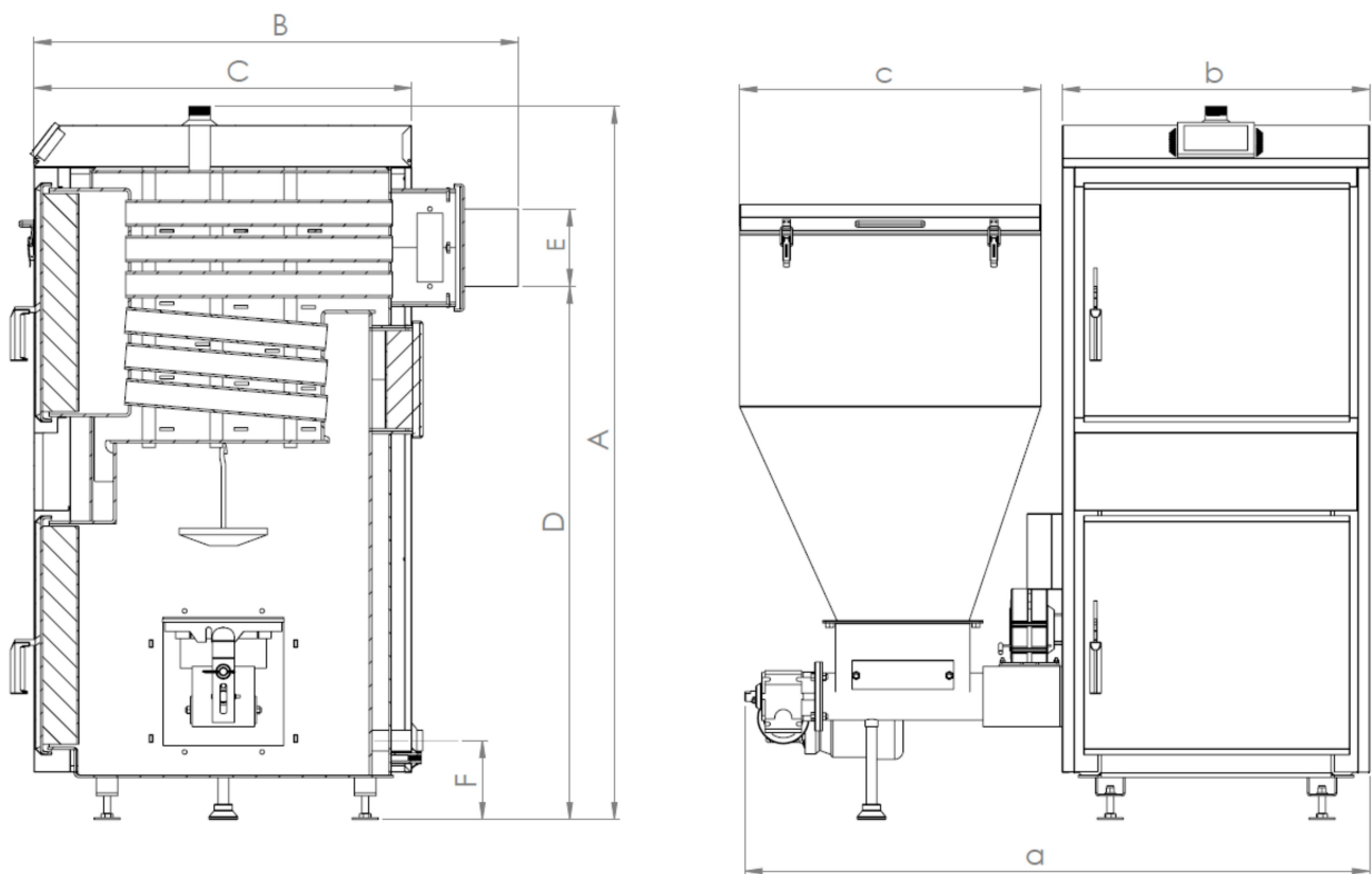
Rys. 3. Wymiary gabarytowe kotła „RETOP”
